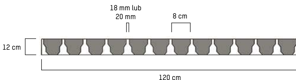
Podłoga szczelinowa dla świń w przekroju
